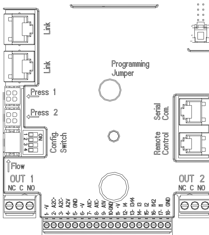
Figura 3: Conessioni
