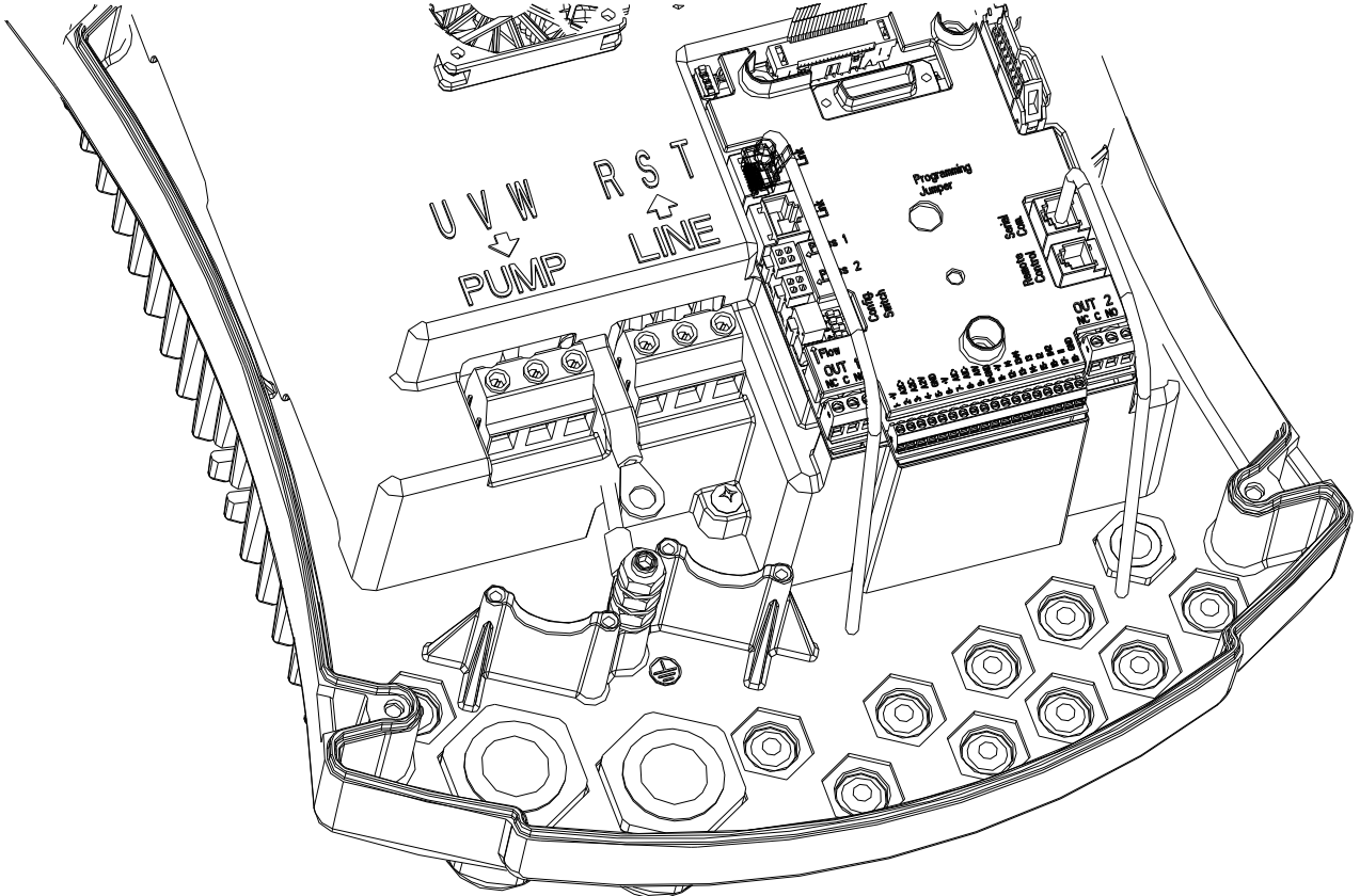
Resim 1: Elektrik Bağlantıları
