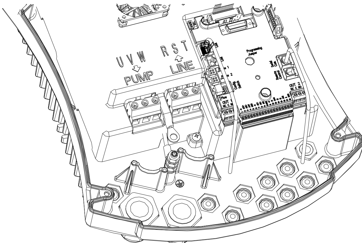
Figura 1: Conexiuni Electrice
