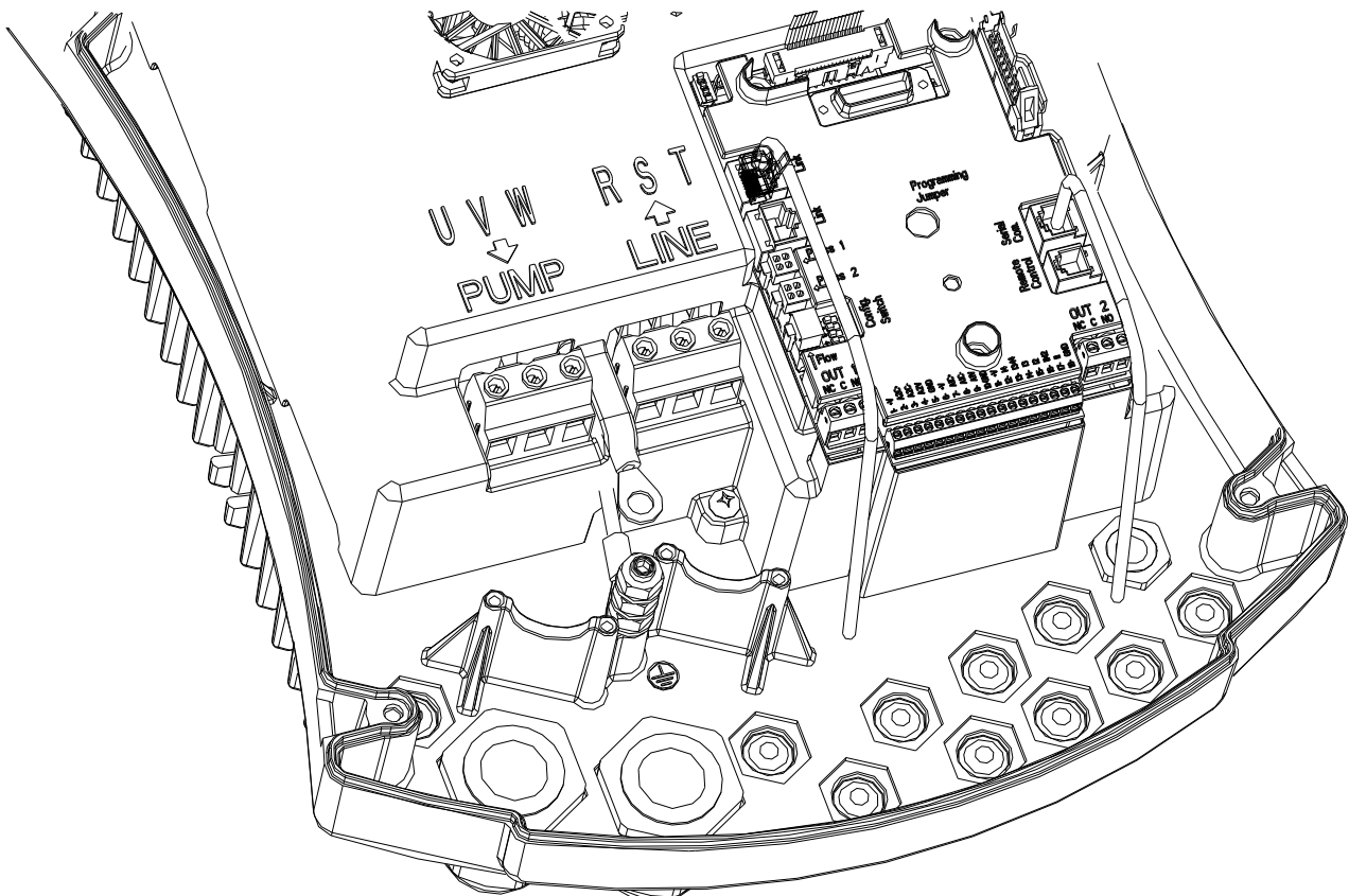
Fig. 1: Elanslutning
