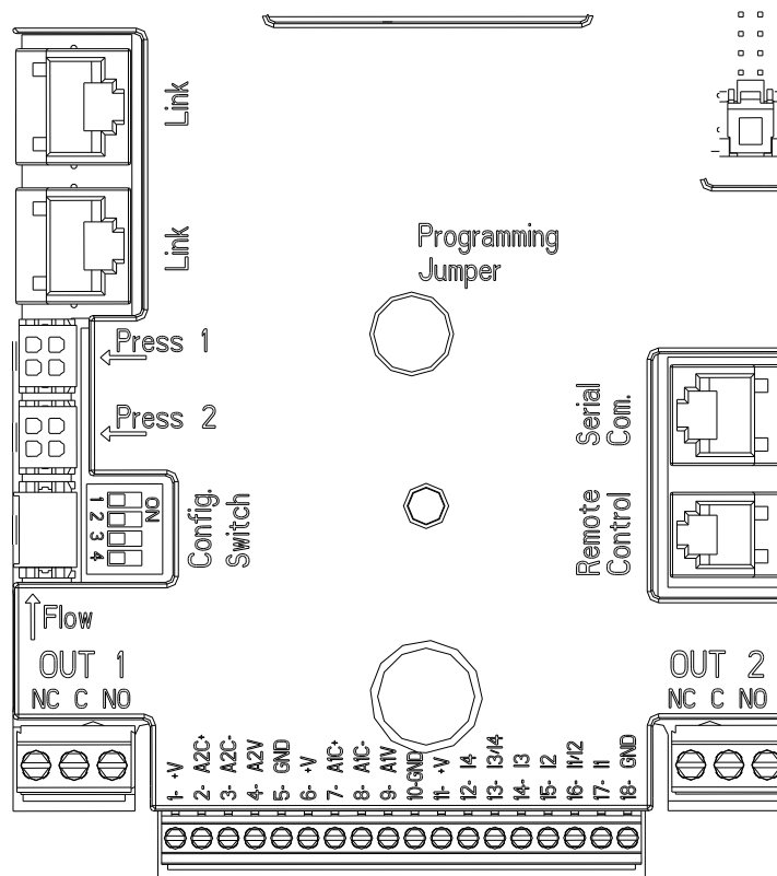
Figura 3: Conexiones
