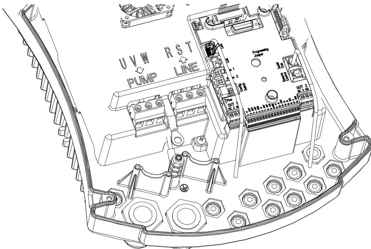
Σχήμα 1: Ηλεκτρική Συνδεσμολογία
