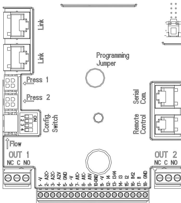
Σχήμα 3: Συνδέσεις
