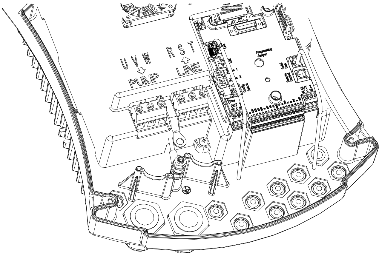
Figure 1: Connexions électriques
