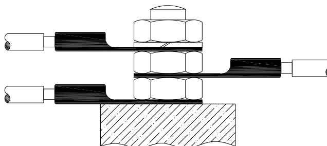
Abbildung 2: Erdungsanschluss
