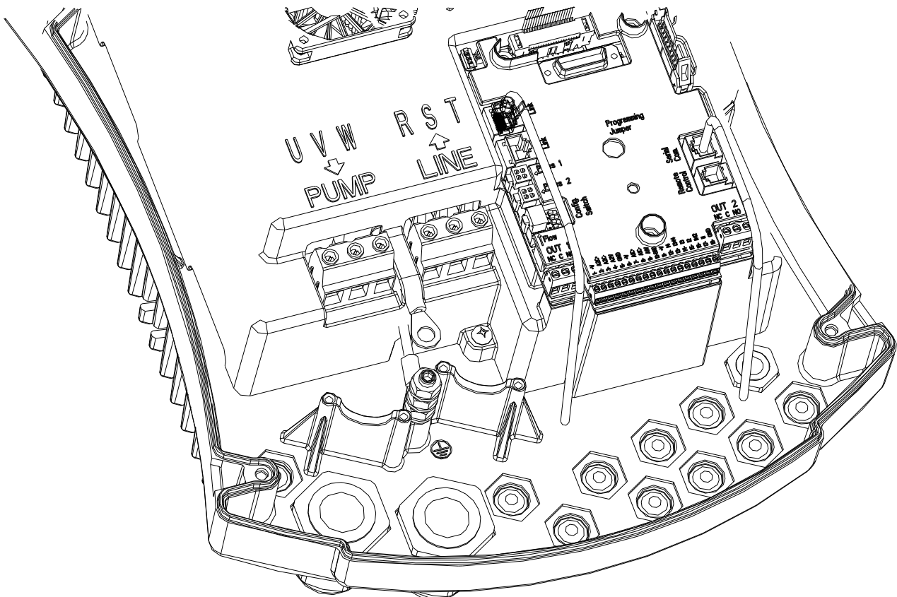
Figura 1: Conexiones eléctricas
