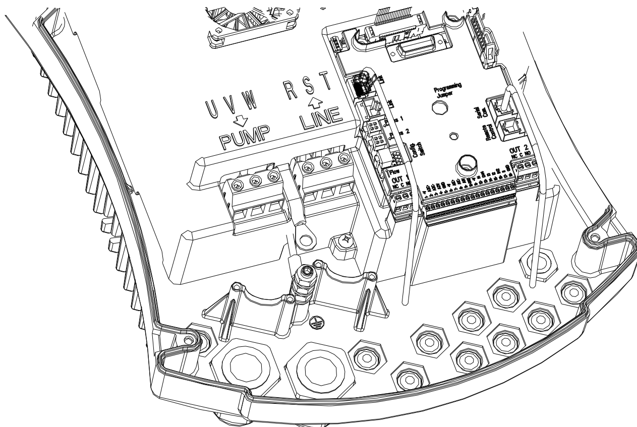
Abbildung 1: Elektroanschlüsse
