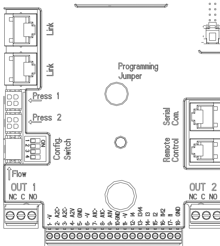
Slika 3: Priključki
